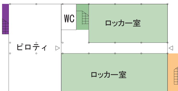
7号館1階 498㎡ S=1/300
